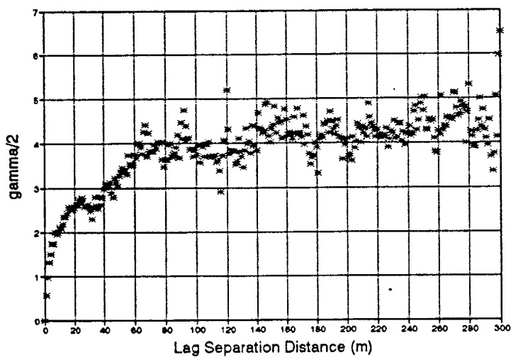
Direction N90E
