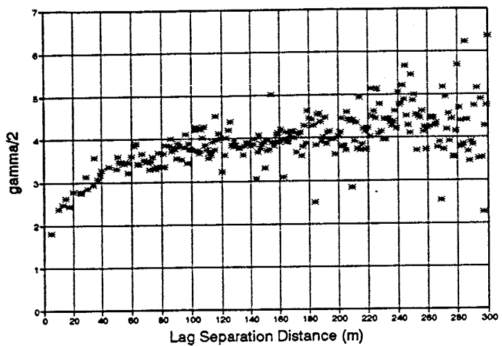
Direction N45E
